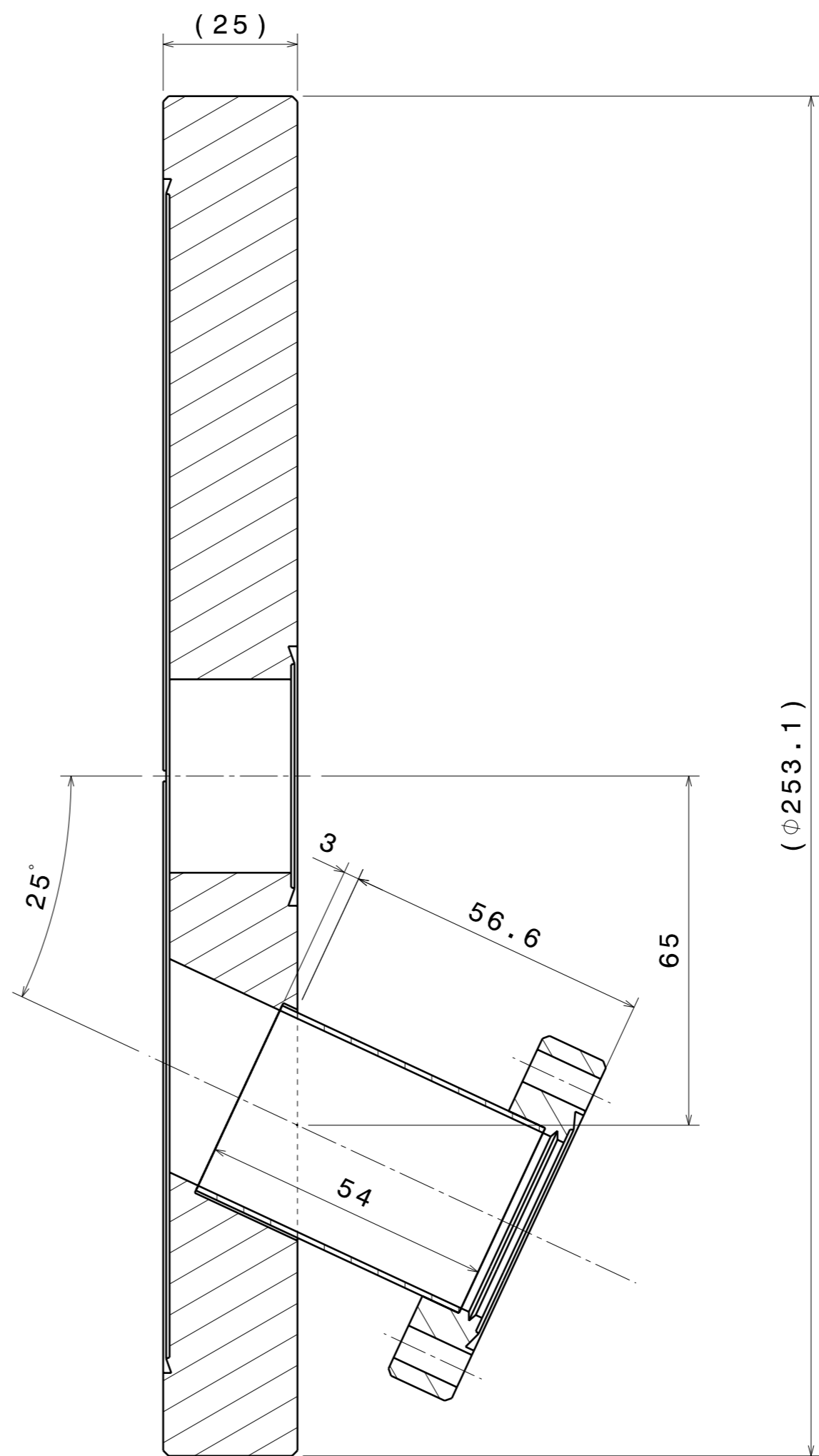
Vista in sezione A-A
