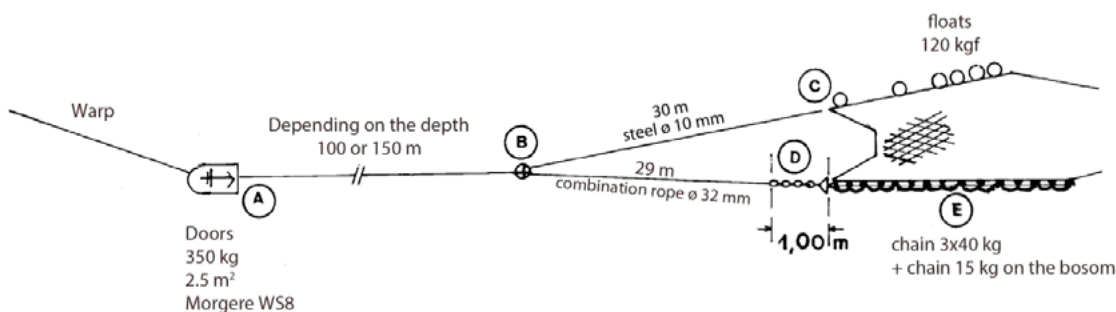
Figura 1 – Dettaglio dell’armamento richiesto per divergenti, calamenti e rete.
