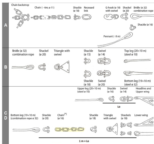
Figura 2 - Ulteriori dettagli relativi alle sezioni A, B, C, e D di figura 1.
