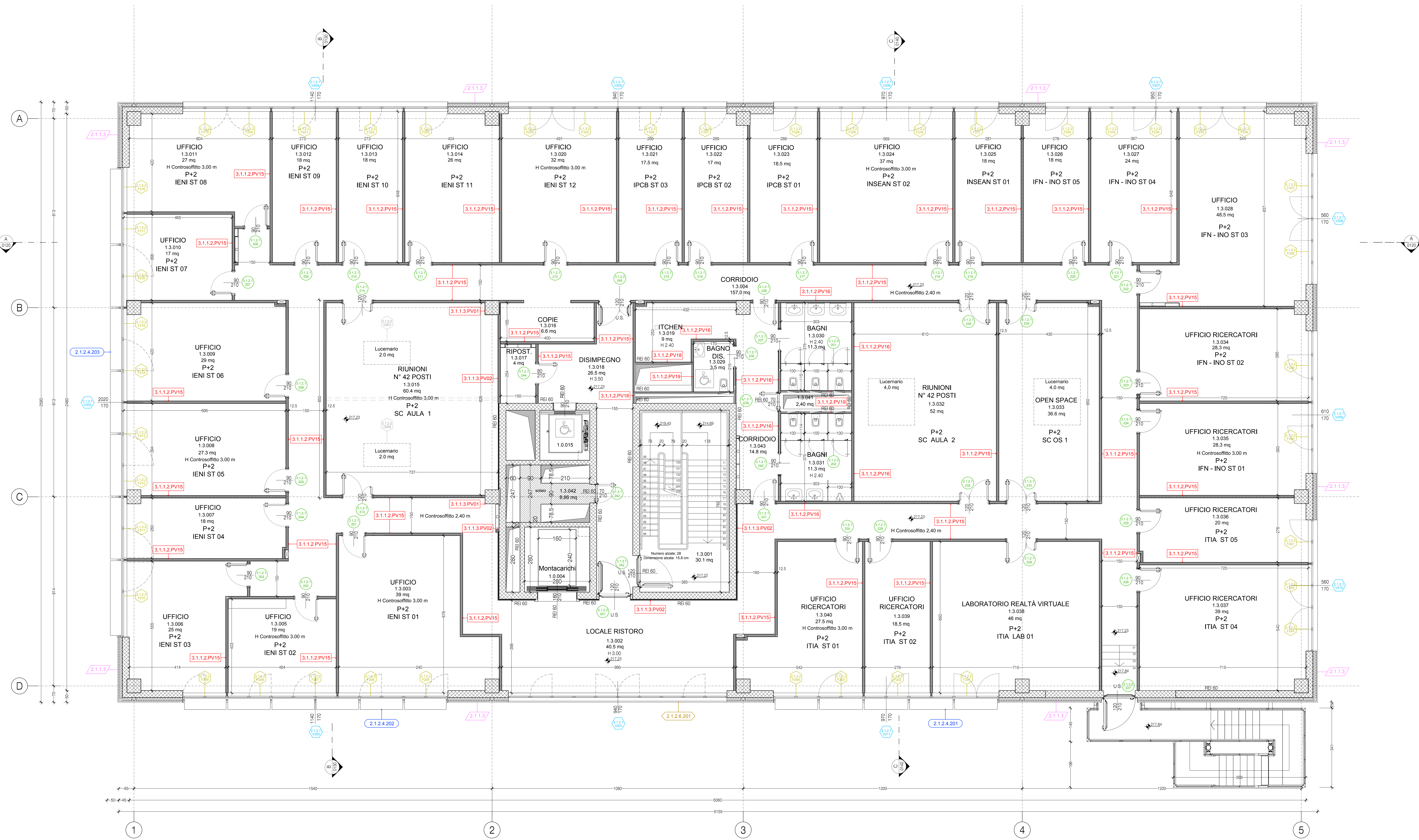
PIANTA LIVELLO +2 +217.23
